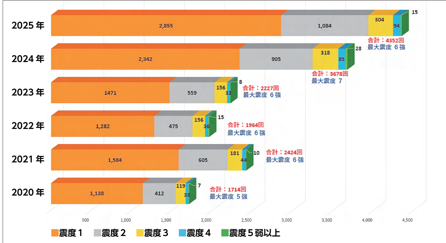
■年度別地震発生回数（震度1以上） ※2025 年は 12 月 14 日まで
