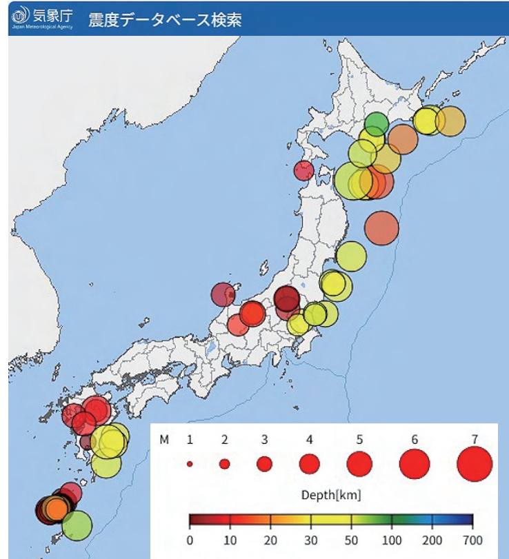
■2025 年の地震 震度4以上
