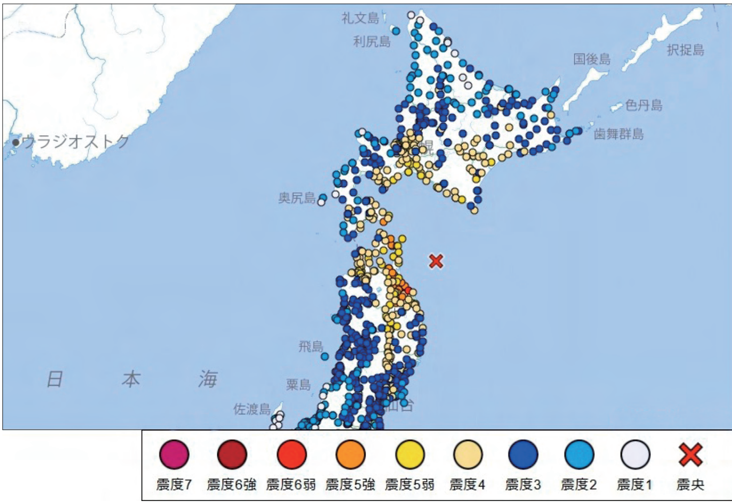
■青森県東方沖地震震度分布（2025 年 12 月 8 日）
